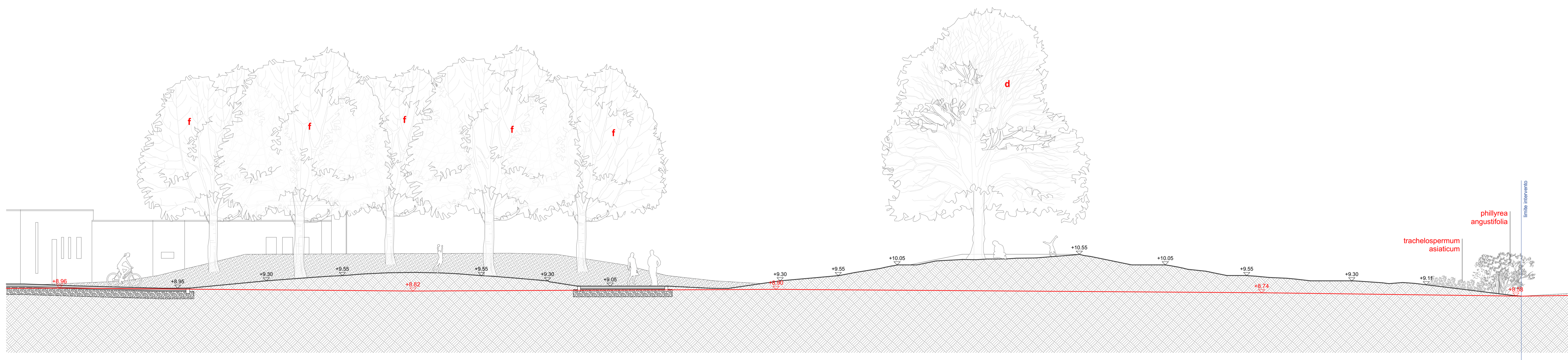
SEZIONE F-F' - scala 1:100
