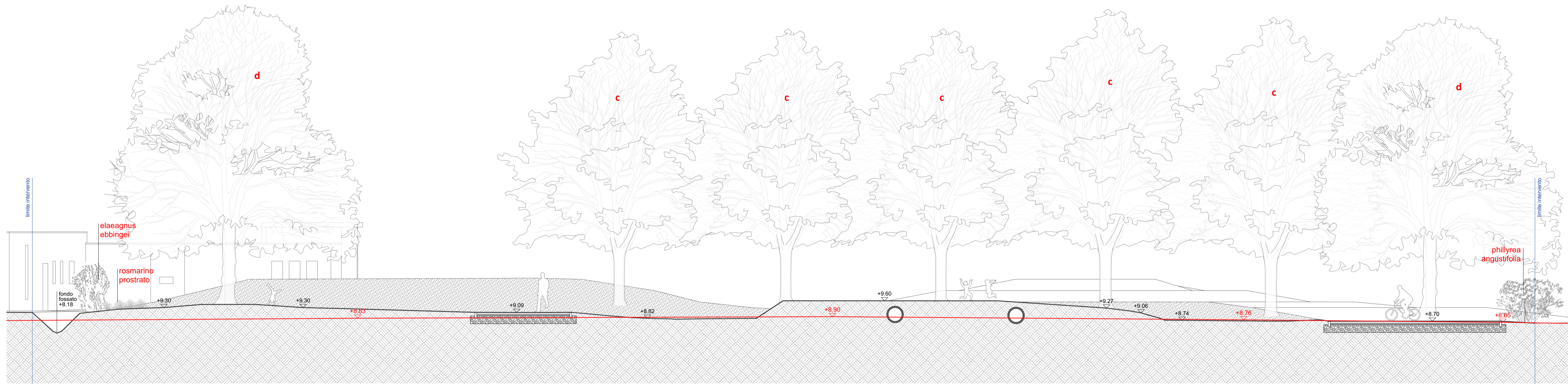
SEZIONE E-E' - scala 1:100
