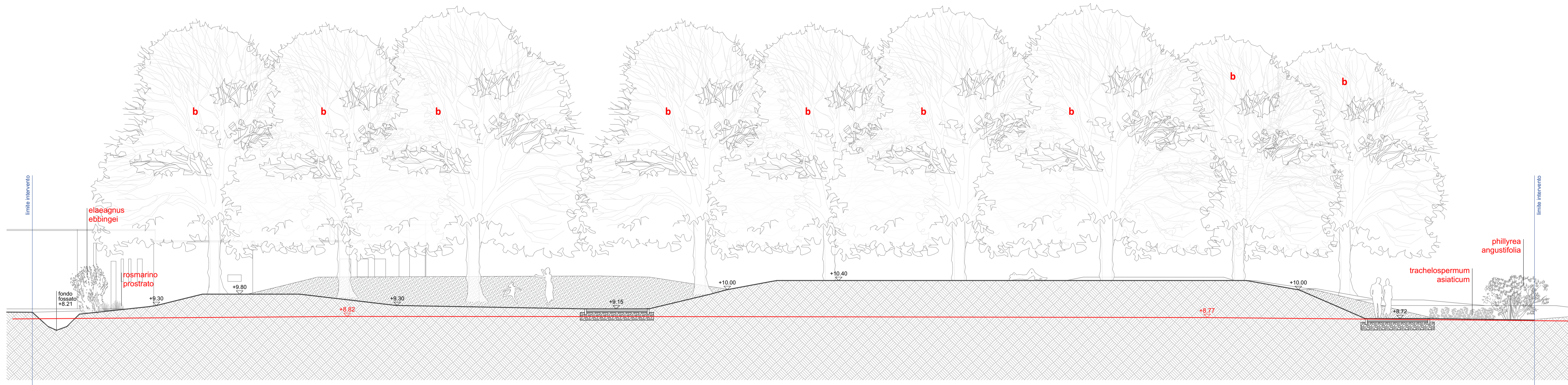
SEZIONE D-D' - scala 1:100
